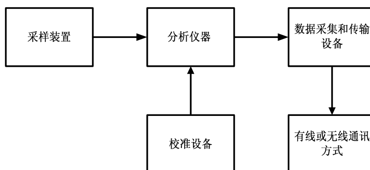
图1 点式连续监测系统组成示意图
