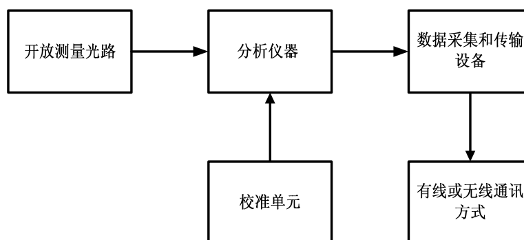
图2 开放光程连续监测系统组成示意图
